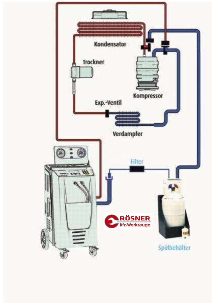
Bild 4 Schematische Darstellung einer kompletten Spülung mit direktem Anschluss über Anschlussadapterplatte am abgeklemmten Kompressor unter Zuhilfenahme von R134A und Spüladapter anstelle des Expansionsventils.
